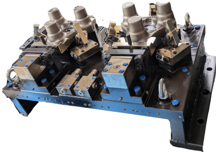
PPC Hyd. Fixture
